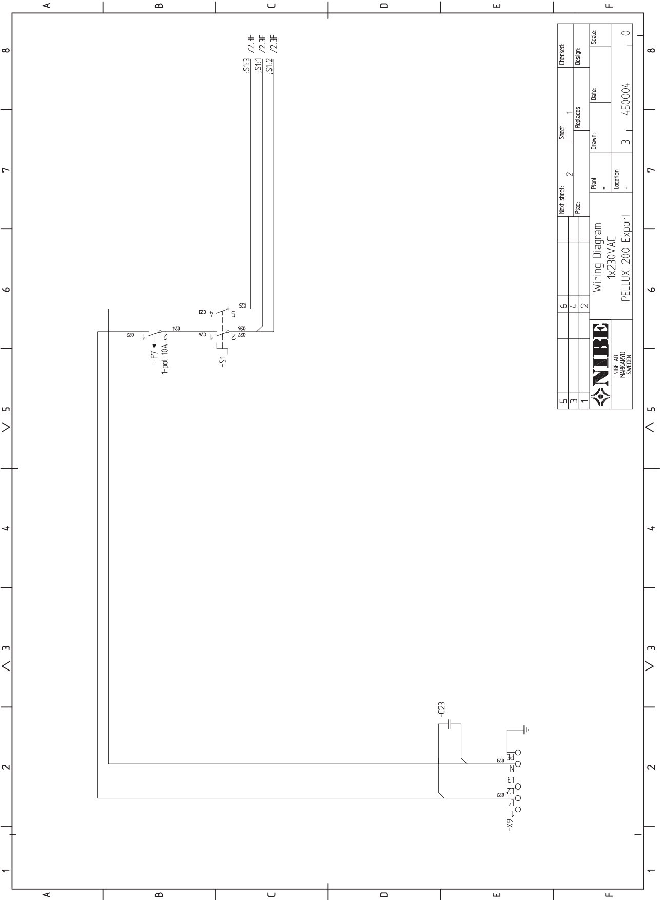
El-skema for strømforsyning til PELLUX 200
